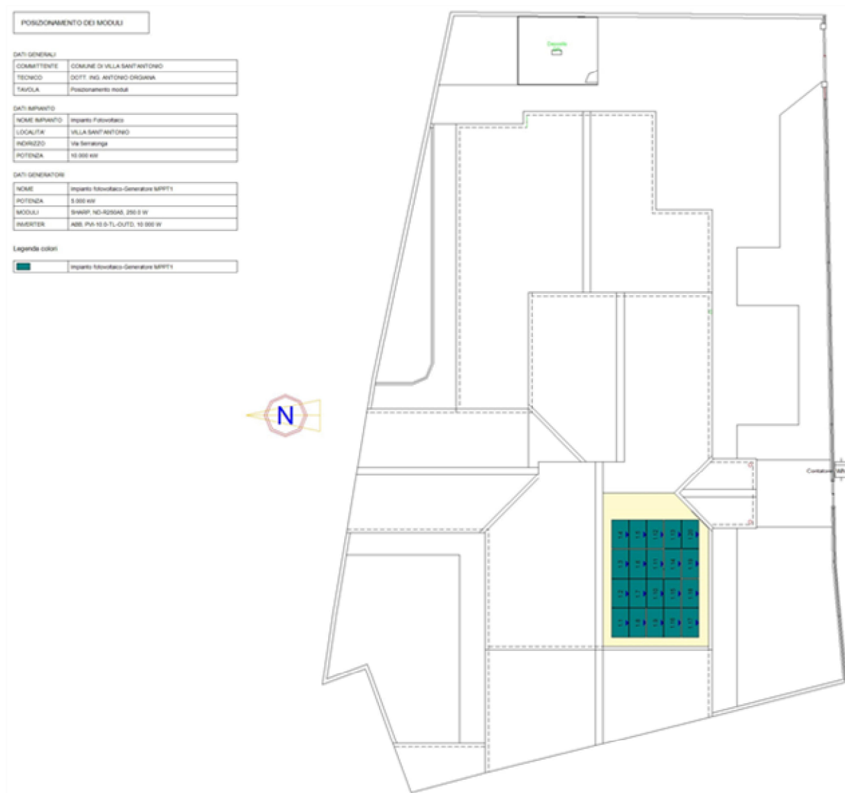
Fig. 4: Posizionamento dei moduli del generatore MPPT Impianto fotovoltaico-Generatore MPPT1
