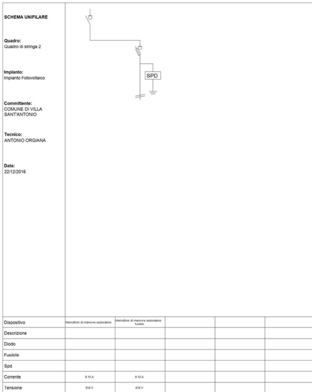
Fig. 9: Schema unifilare quadro "Quadro di stringa 2"
