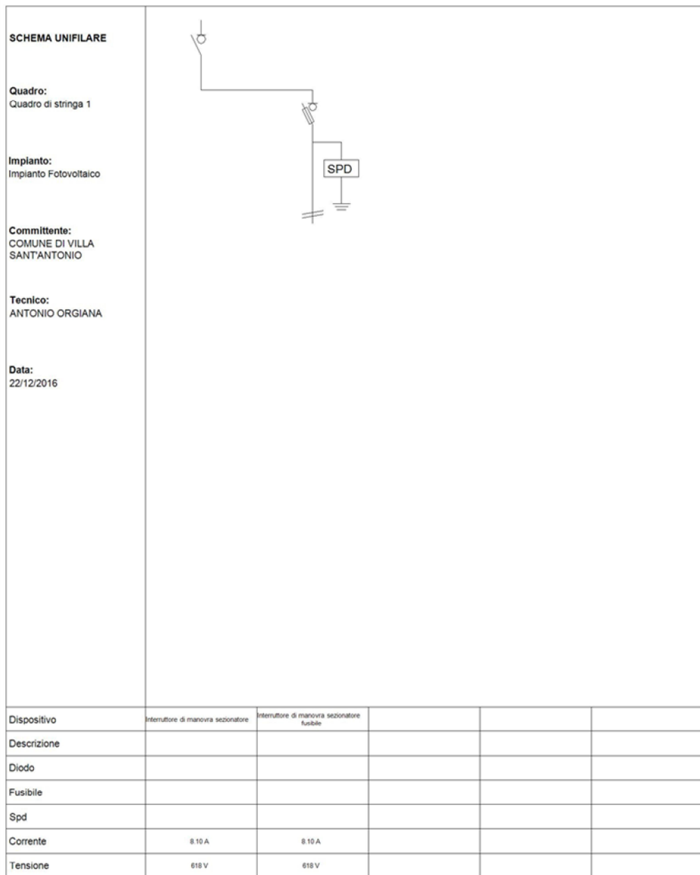
Fig. 8: Schema unifilare quadro "Quadro di stringa 1"
