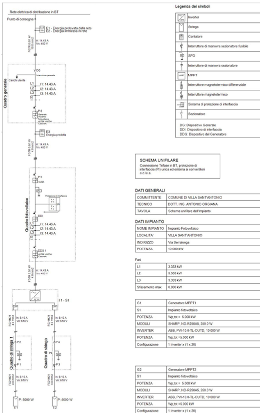
Fig. 10: Schema elettrico unifilare dell'impianto
