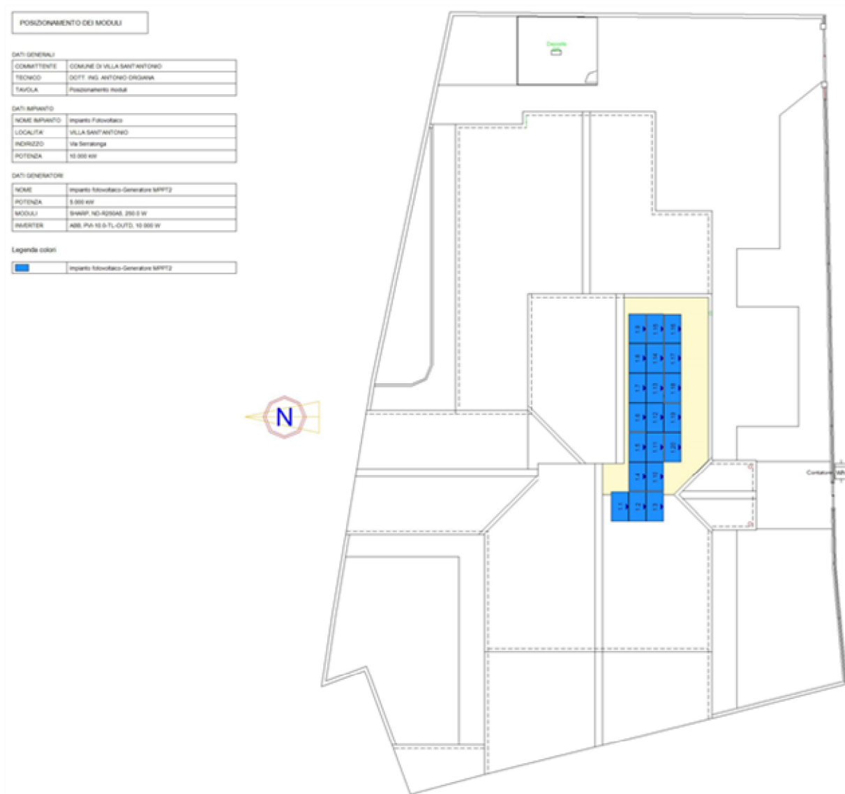
Fig. 5: Posizionamento dei moduli del generatore MPPT Impianto fotovoltaico-Generatore MPPT2
